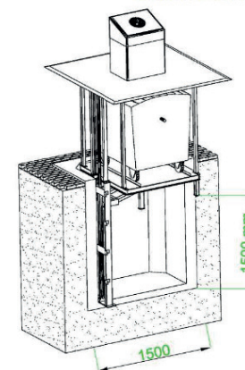
DŹWIGNIK oraz KOMORA ŻELBETONOWA
